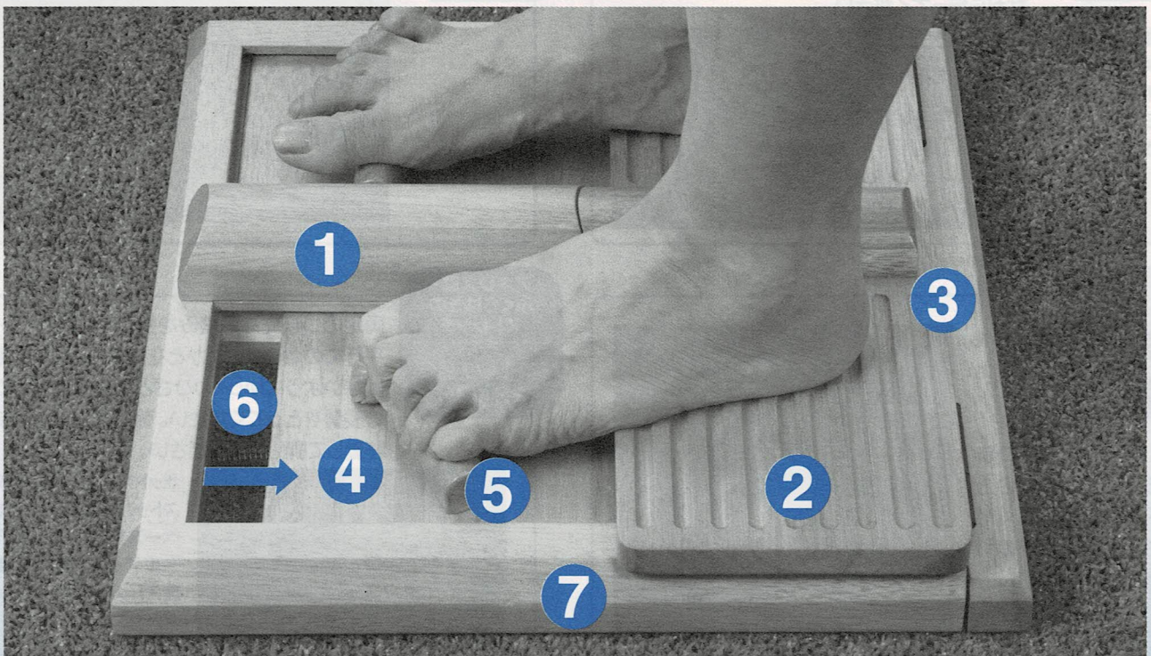
①足踏み ②ヒールベース ③角度ストッパー ④スライドベース ⑤フック ⑥パネ ⑦ボディ
